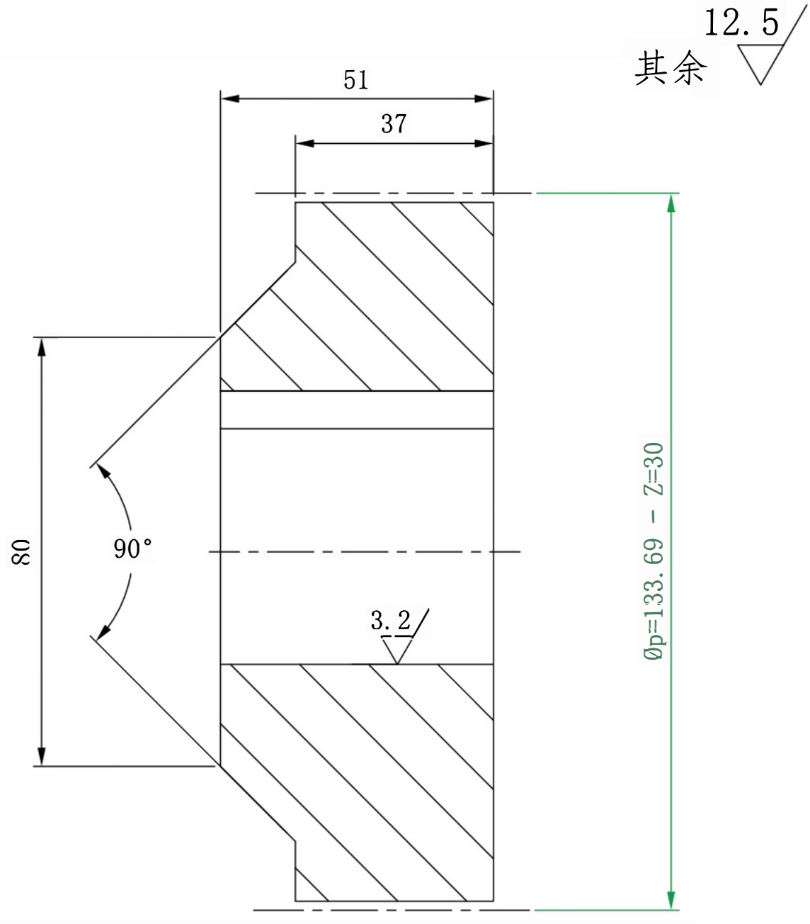
截面 A-A
