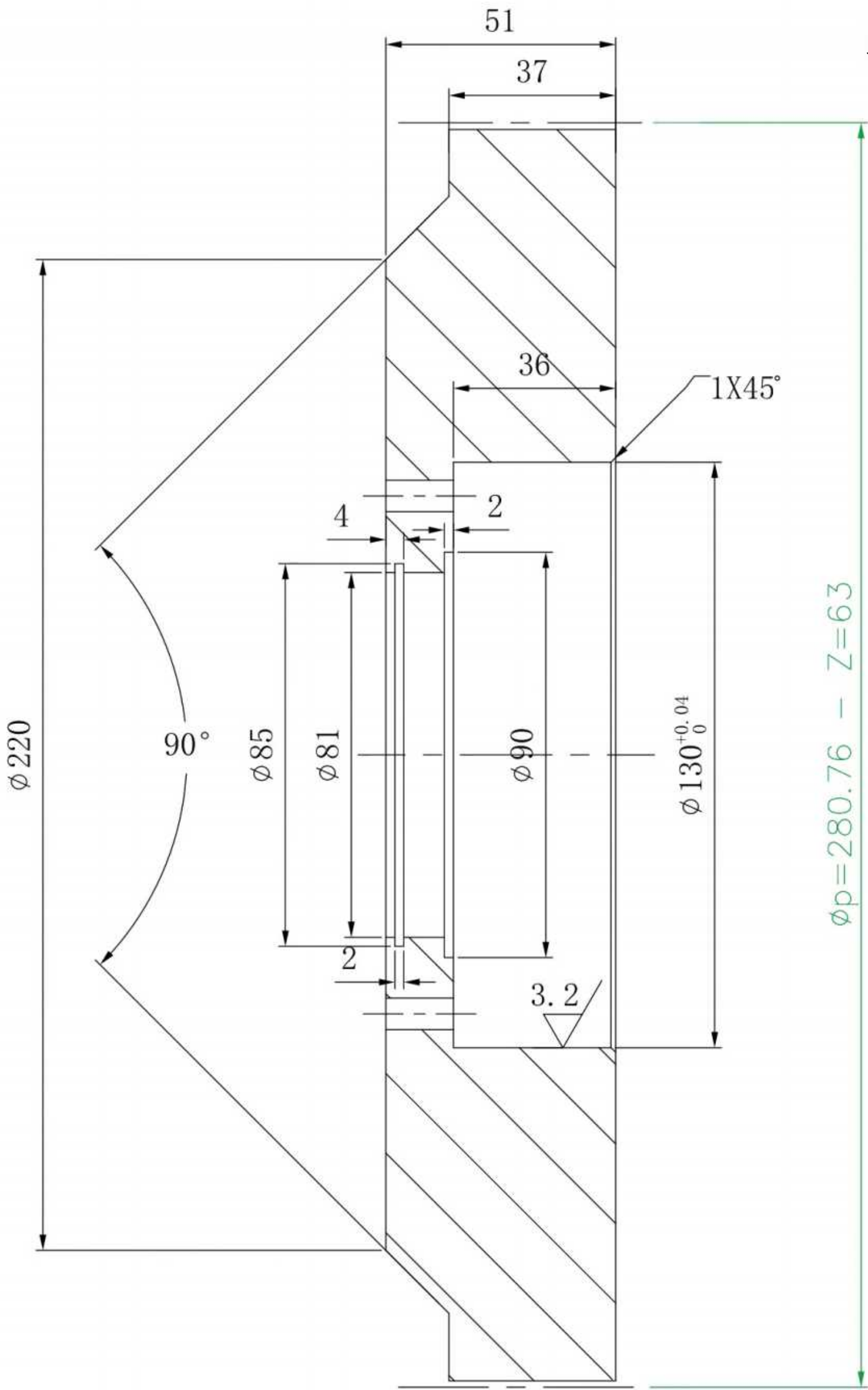
截面 A-A
