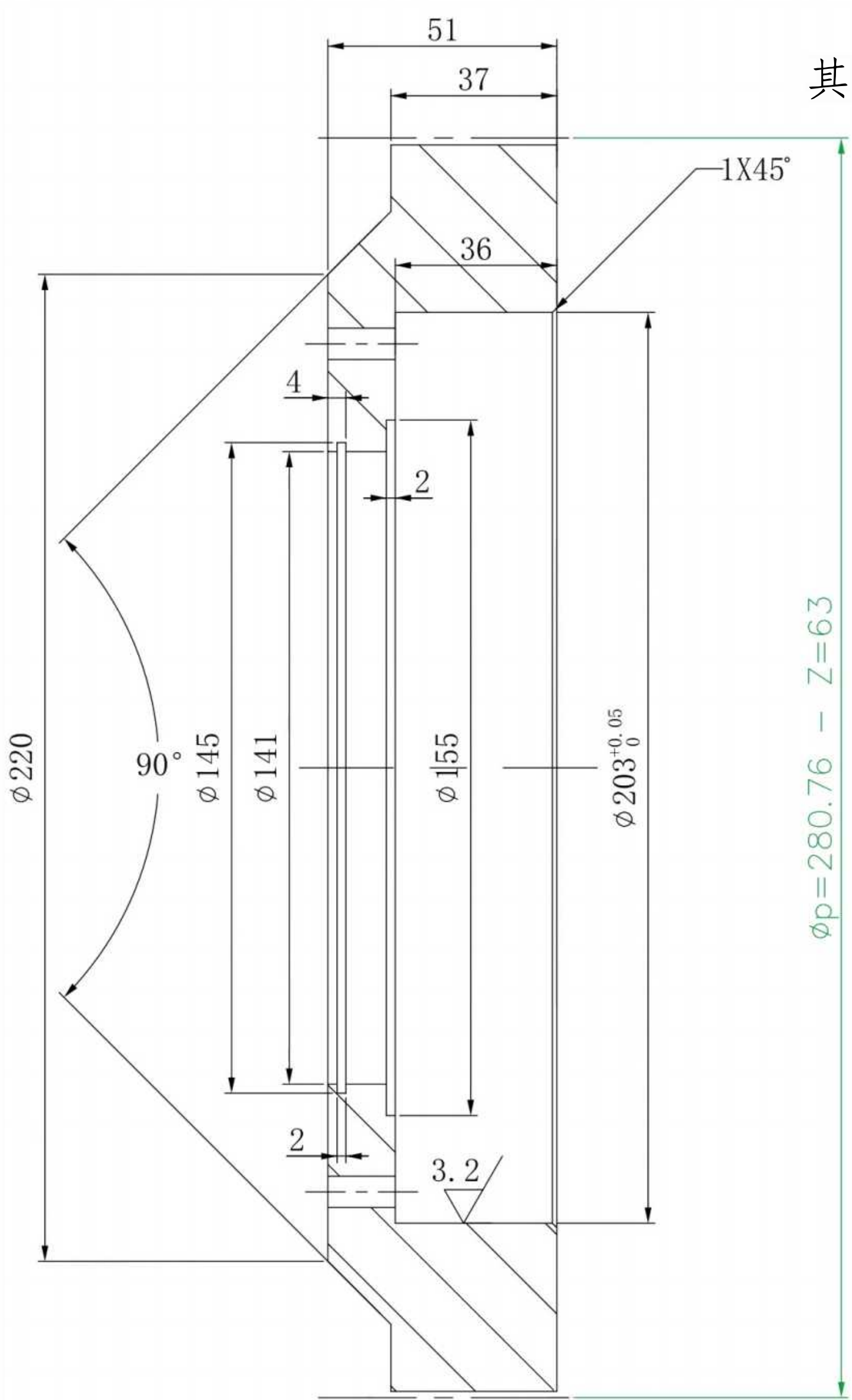
截面 A-A
