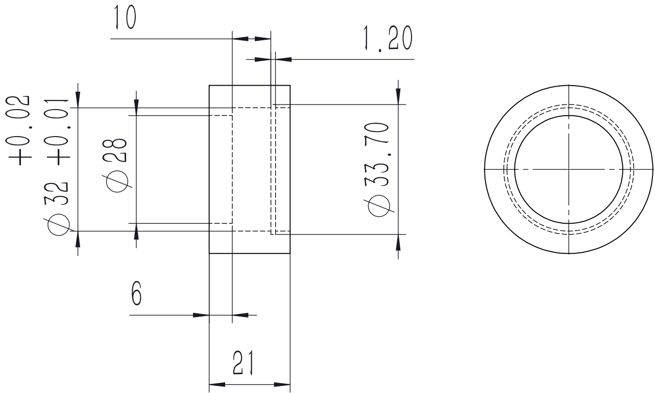
人字齿M5, 28齿
