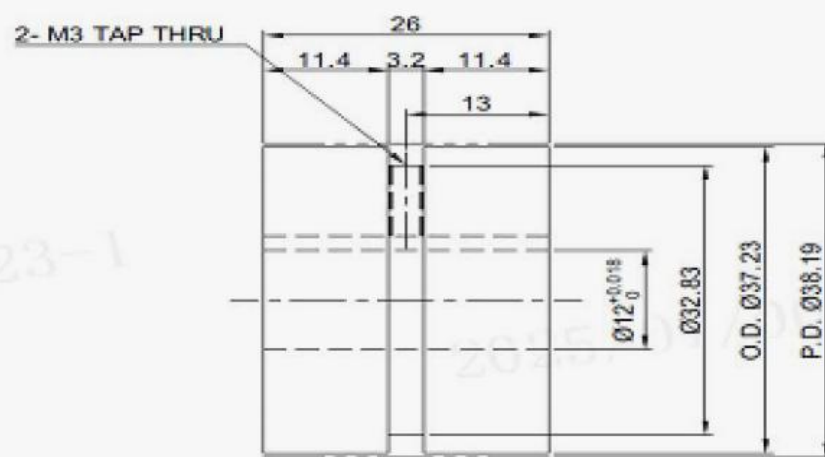
人字齿5M 24齿
