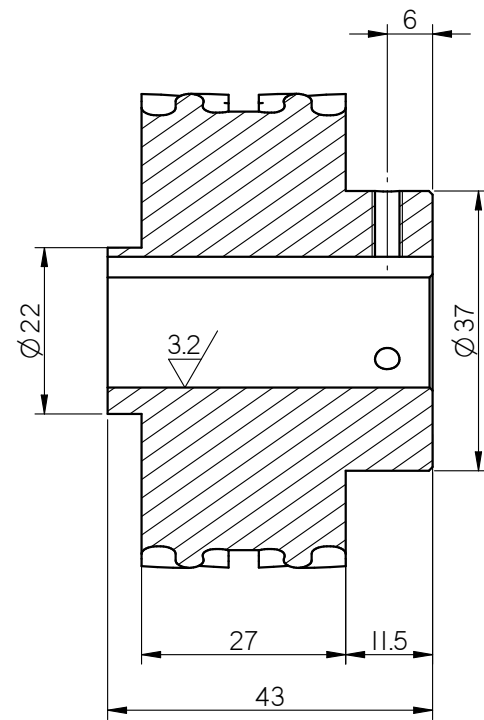
剖面 A-A
