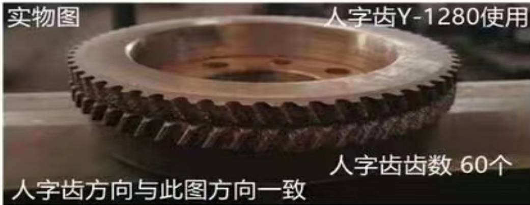
人字齿带轮#2
