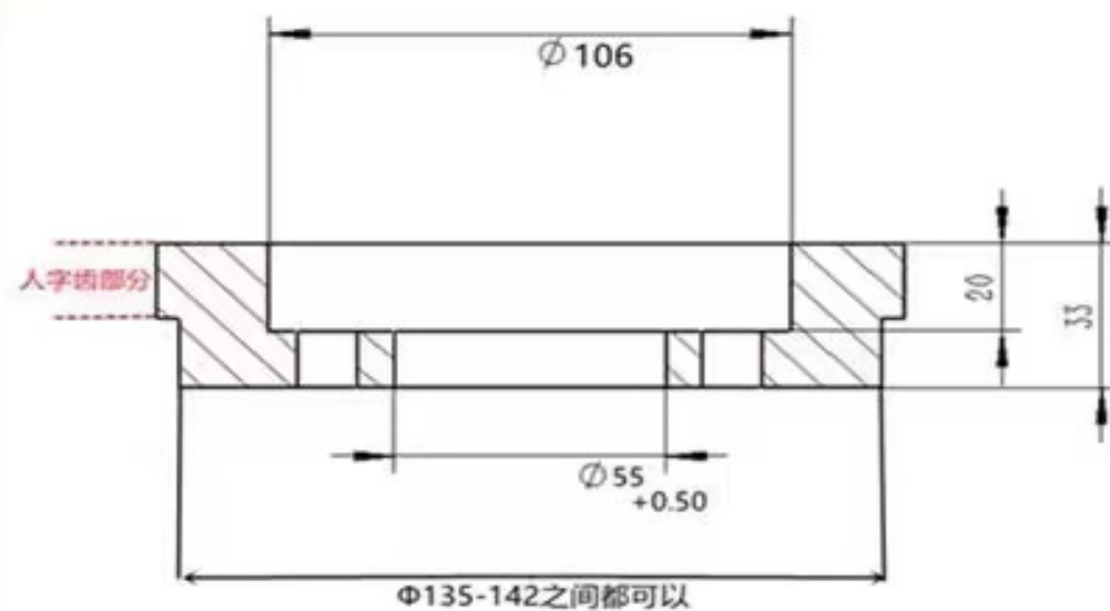
人字齿带轮#2
