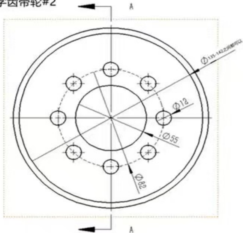
人字齿带轮#2
