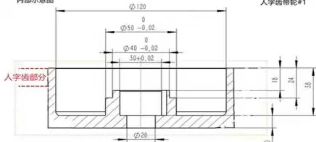
内部示意图
