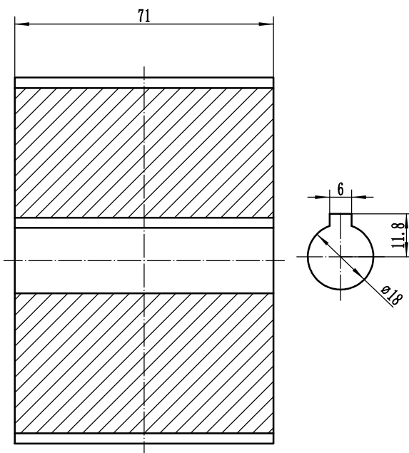
齿形：人字齿E8M 齿数：40齿 材质：6061-T6 本色阳极氧化
