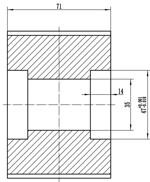
齿形：人字齿E8M 齿数：40齿 材质：6061-T6 本色阳极氧化
