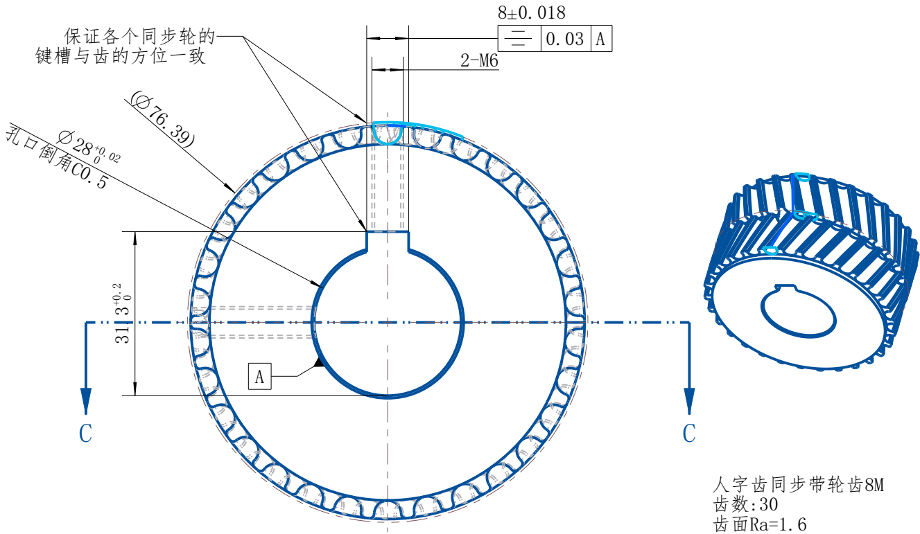
截面 C-C
